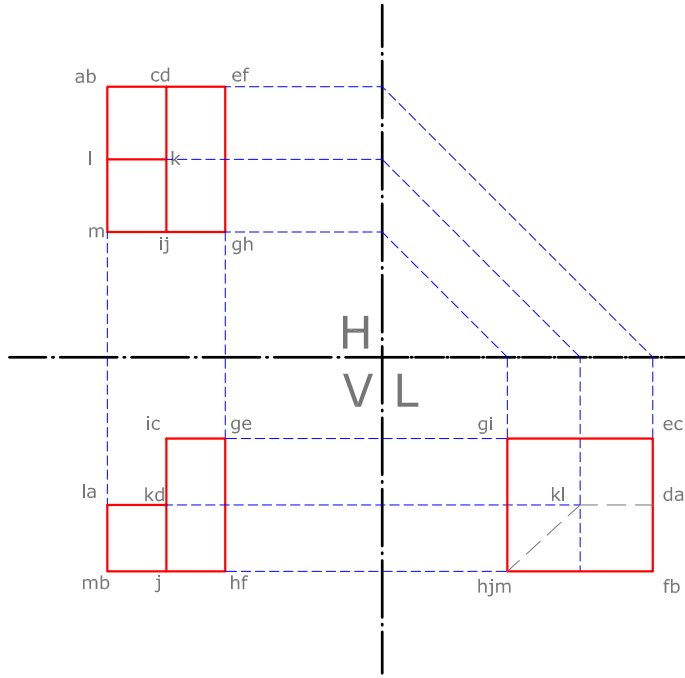
PROYECCIONES ORTOGONALES
