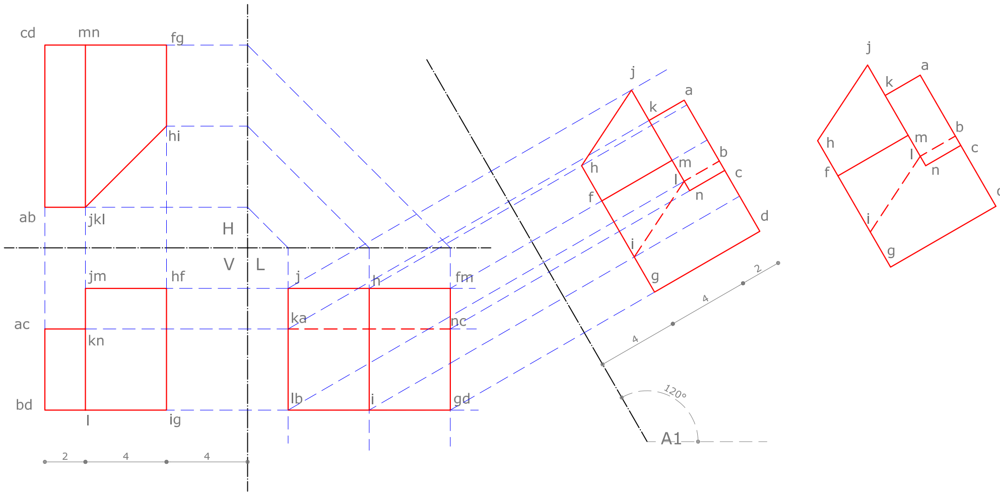
PROYECCION AUXILIAR A_1 \quad A \quad 120^\circ
