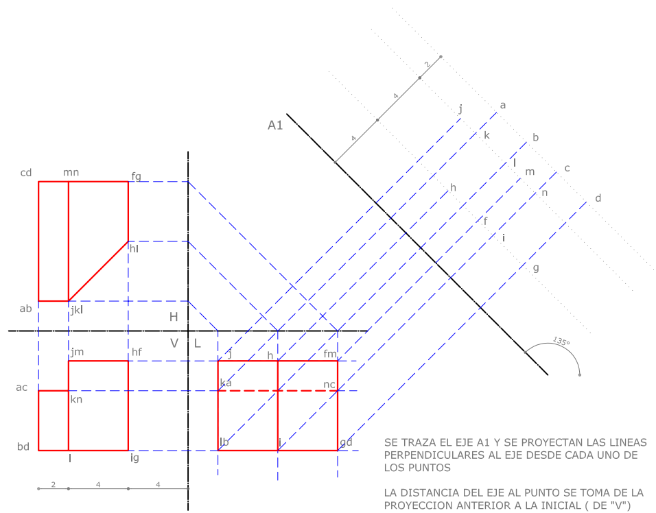
PROYECCION AUXILIAR A1 A 135°
