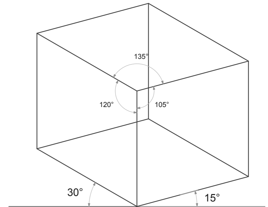
PROYECCION AXONOMETRICA TRIMETRIA
