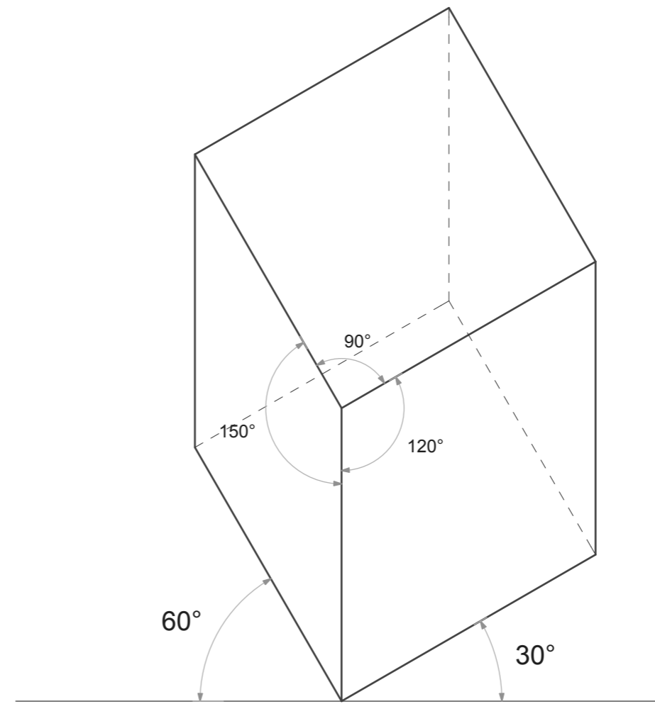
PROYECCION AXONOMETRICA PLANTA OBLICUA TRIMETRIA
