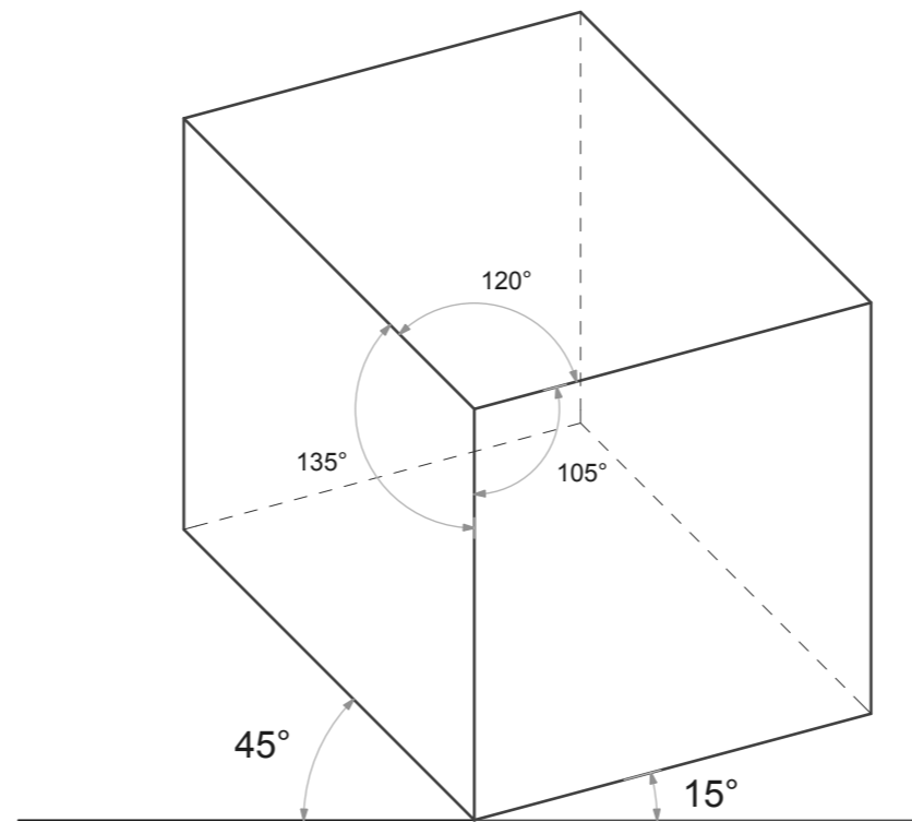
PROYECCION AXONOMETRICA TRIMETRIA
