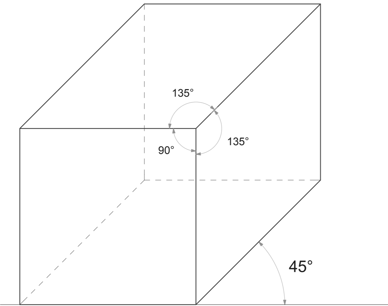
PROYECCION AXONOMETRICA ALZADO OBLICUO (DIBUJO CABALLERO) DIMETRIA
