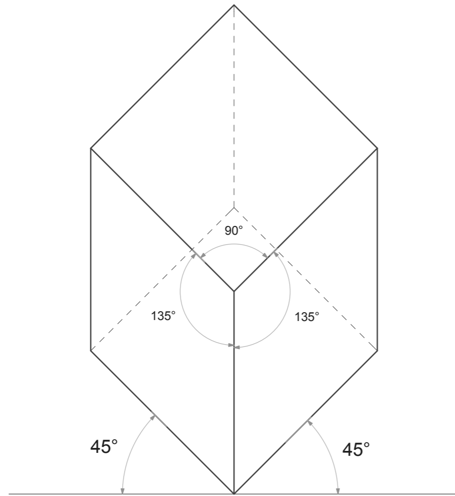
PROYECCION AXONOMETRICA PLANTA OBLICUA (DIBUJO MILITAR) DIMETRIA
