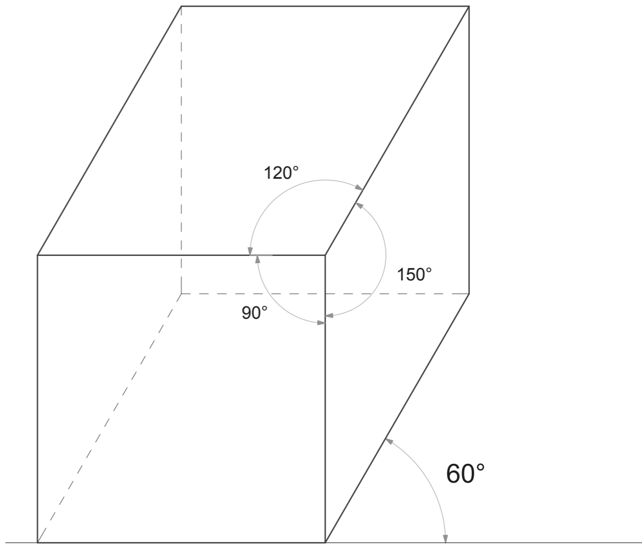
PROYECCION AXONOMETRICA ALZADO OBLICUO (DIBUJO CABALLERO) TRIMETRIA
