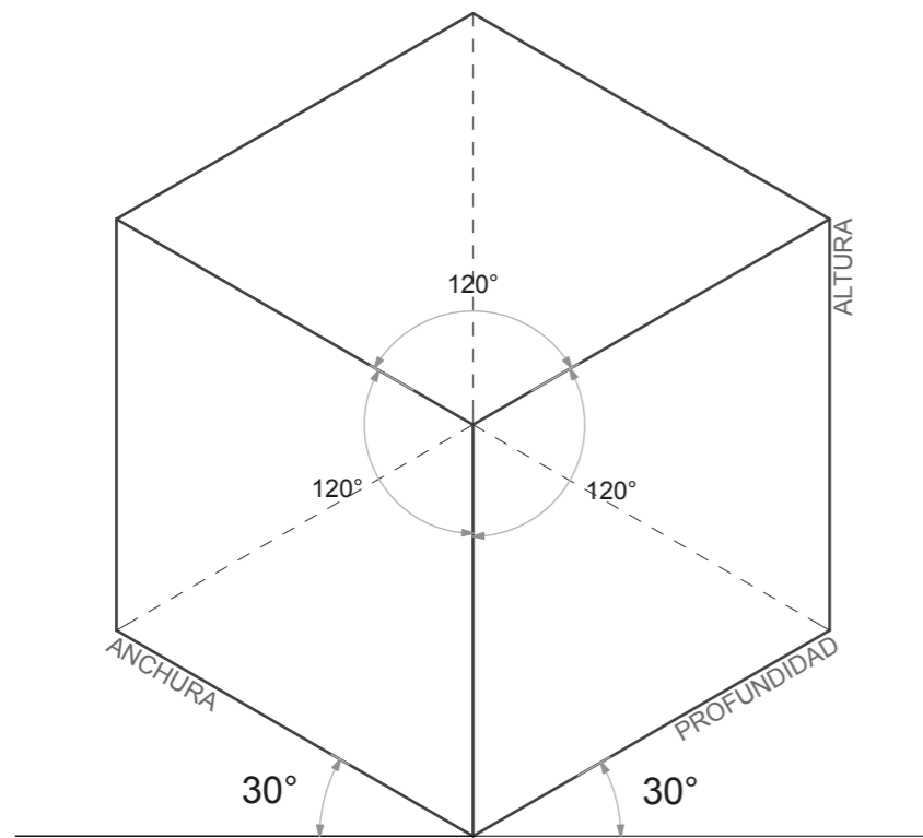
PROYECCION AXONOMETRICA ISOMETRICA
